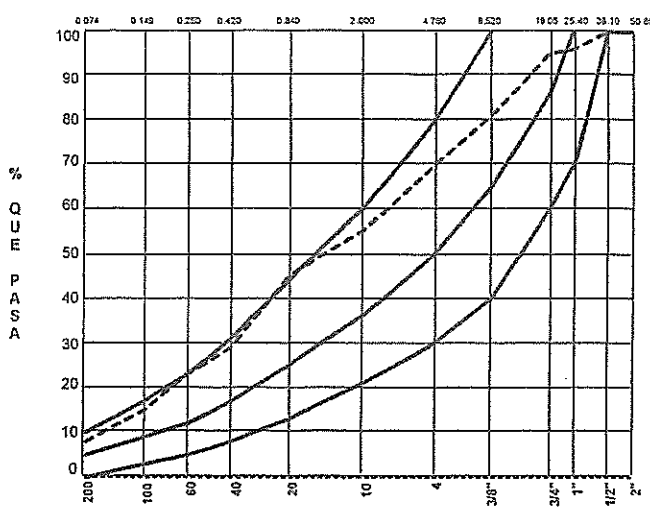
GRAFICA DE COMPOSICIÓN GRANULOMÉTRICA
