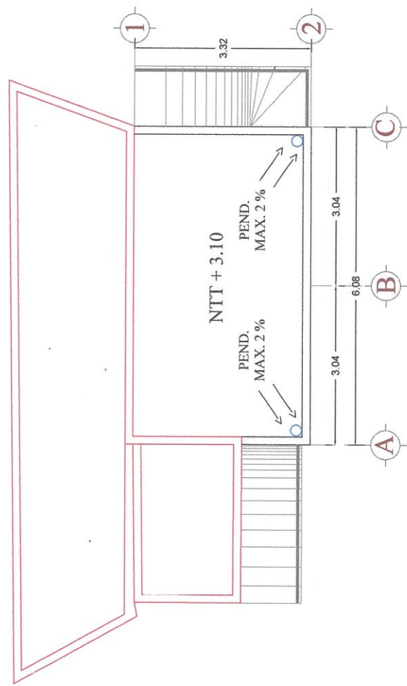
PLANTA DE AZOTEA
